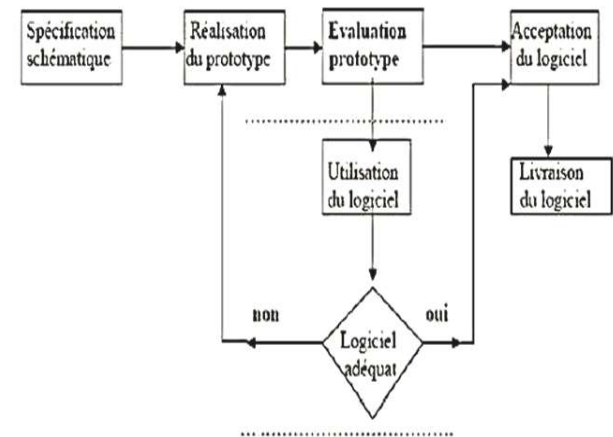
Modèle du cycle de vie par prototypage
