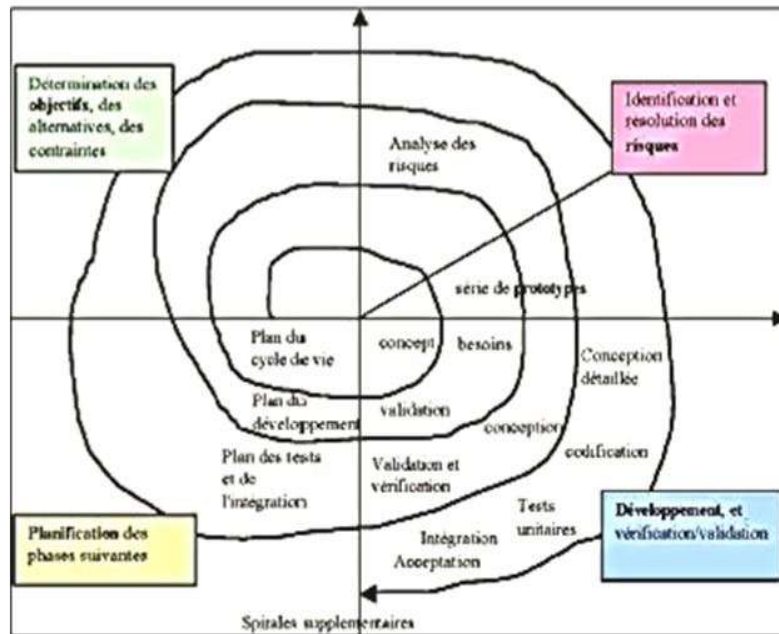
Modèle du cycle de vie en spirale
