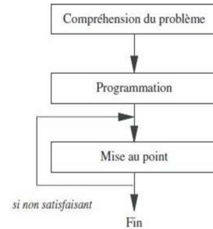
Le modèle du code-and-fix.
